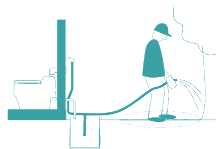
Funktionsschema Ejektortank
